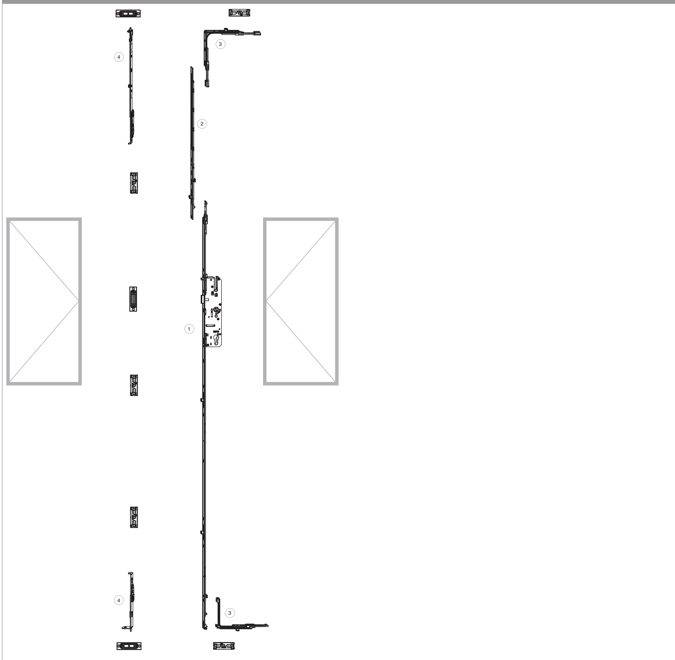
B-TV 2-sashed shootbolt
